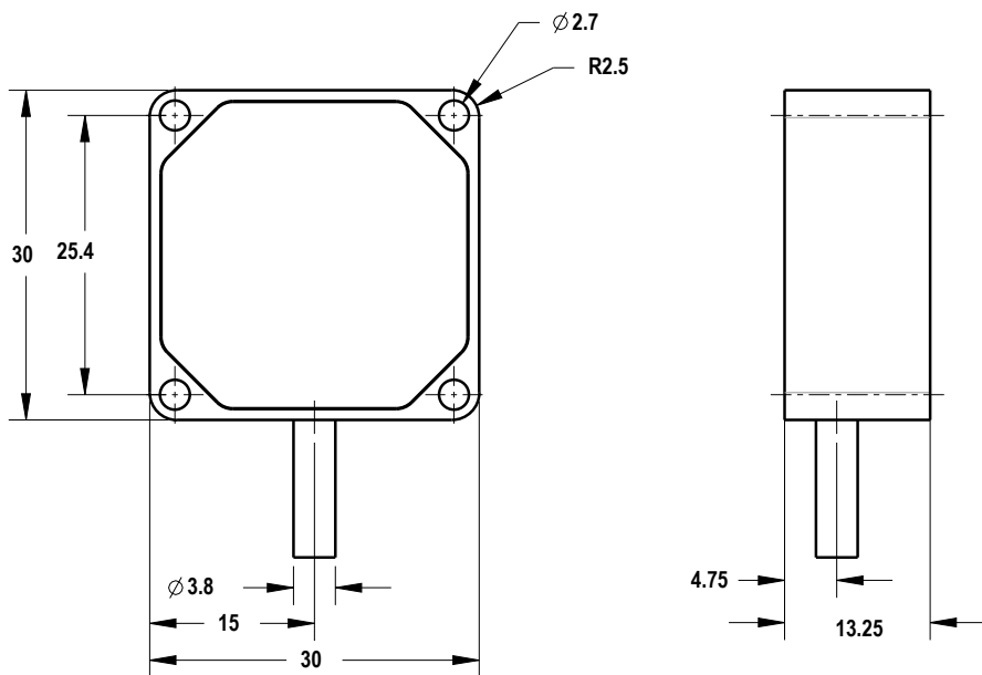
Figura 3. Modelli in acciaio inox
